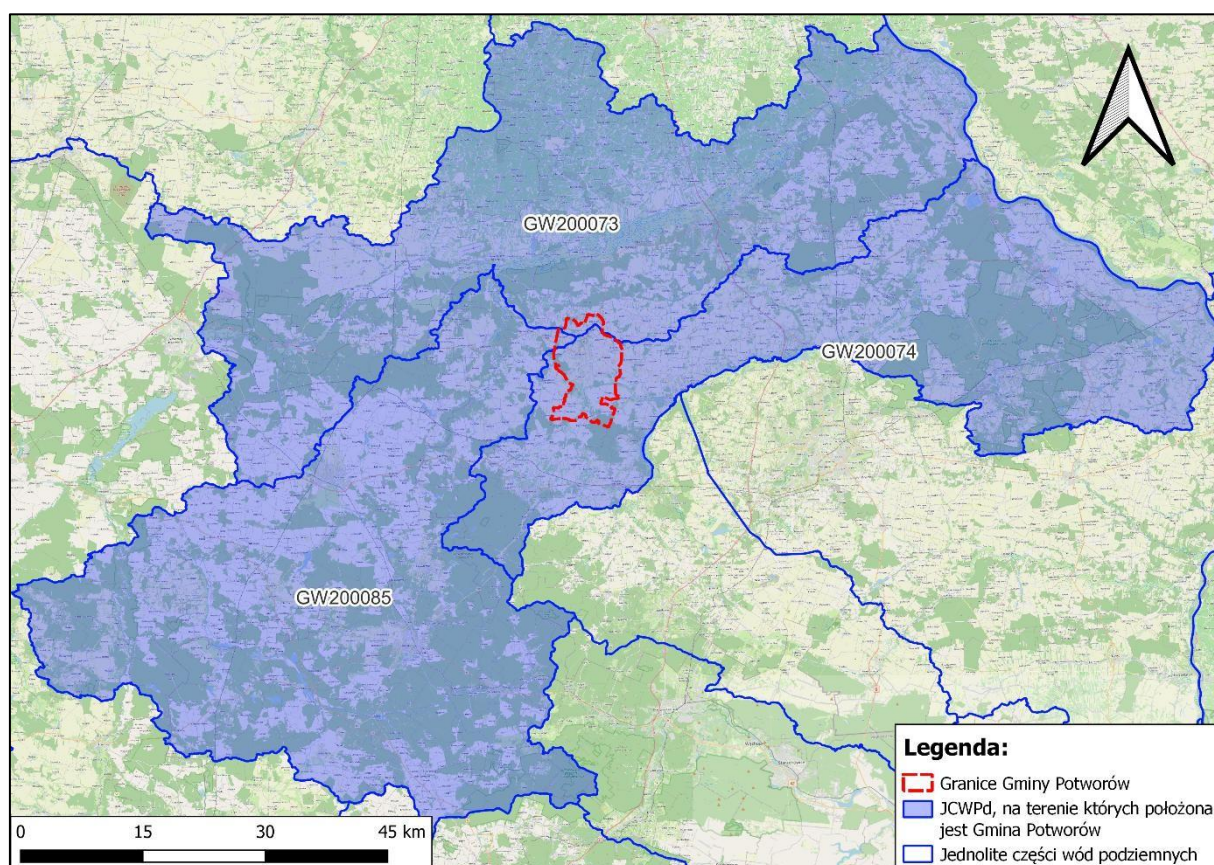
Rysunek 5. Jednostki Części Wód Podziemnych na tle Gminy Potworów
