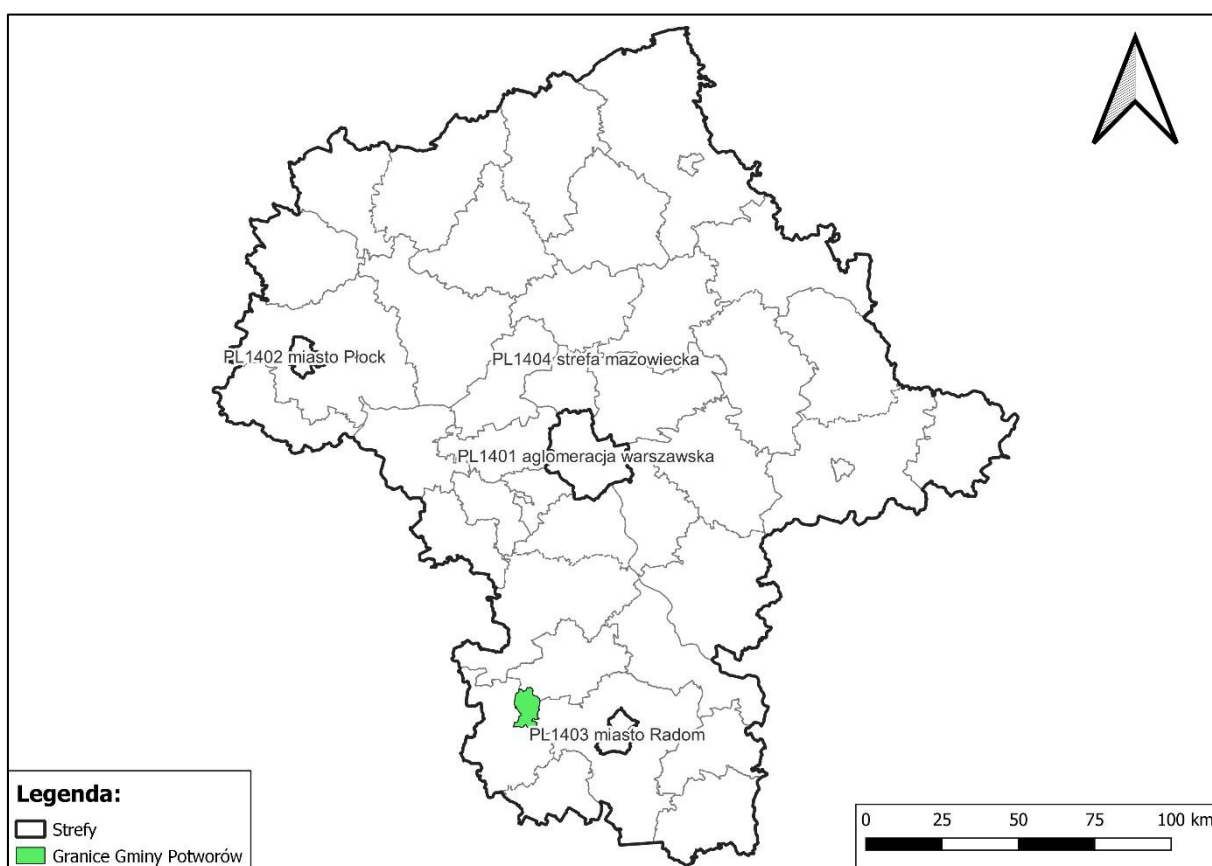
Rysunek 2. Podział województwa mazowieckiego na strefy
