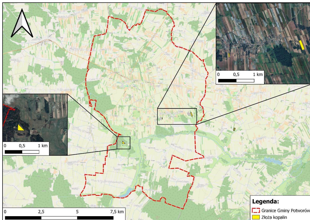
Rysunek 7. Złoża kopalni na tle Gminy Potworów
