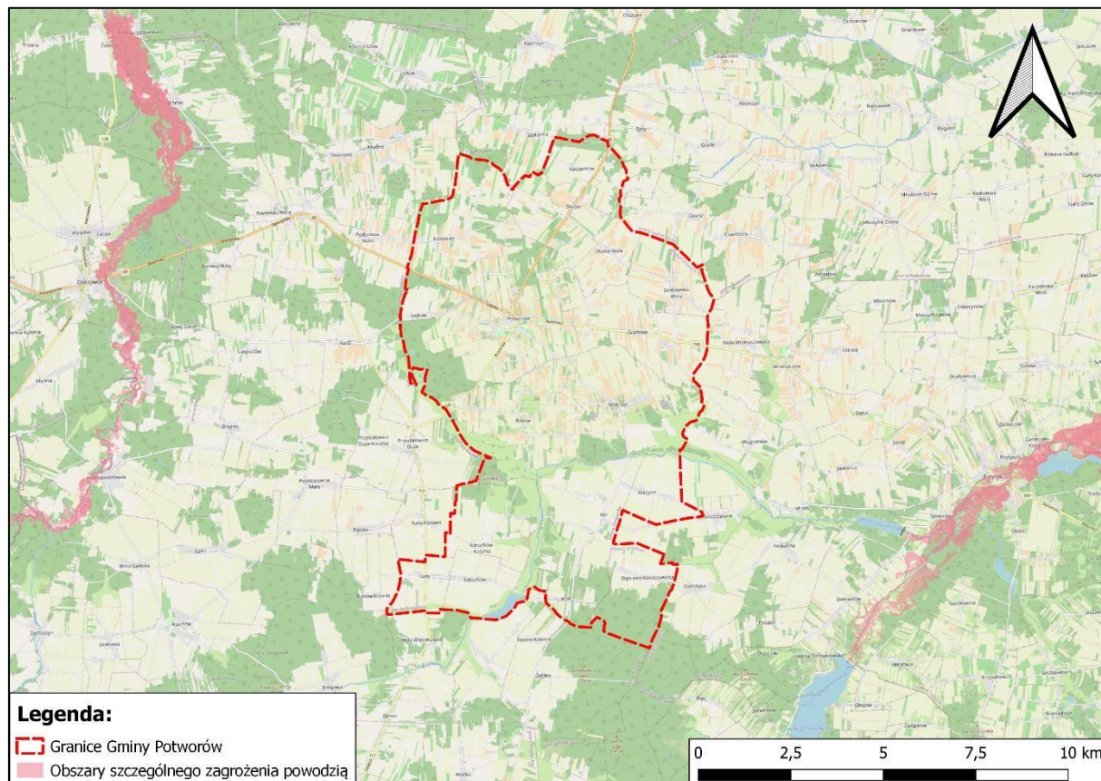
Rysunek 4. Zagrożenie powodziowe na terenie Gminy Potworów
